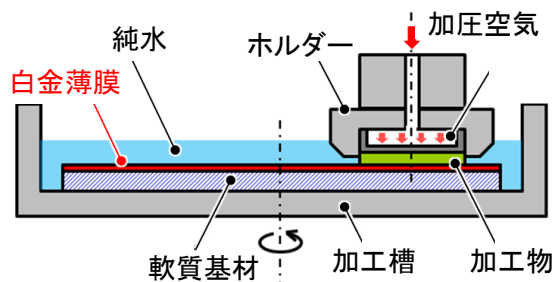
図2 Water-CARE 装置。パッド表面に触媒金属の薄膜が形成されている以外は、通常の研磨装置とほぼ同等。軟質基材は通常の研磨パッド。
